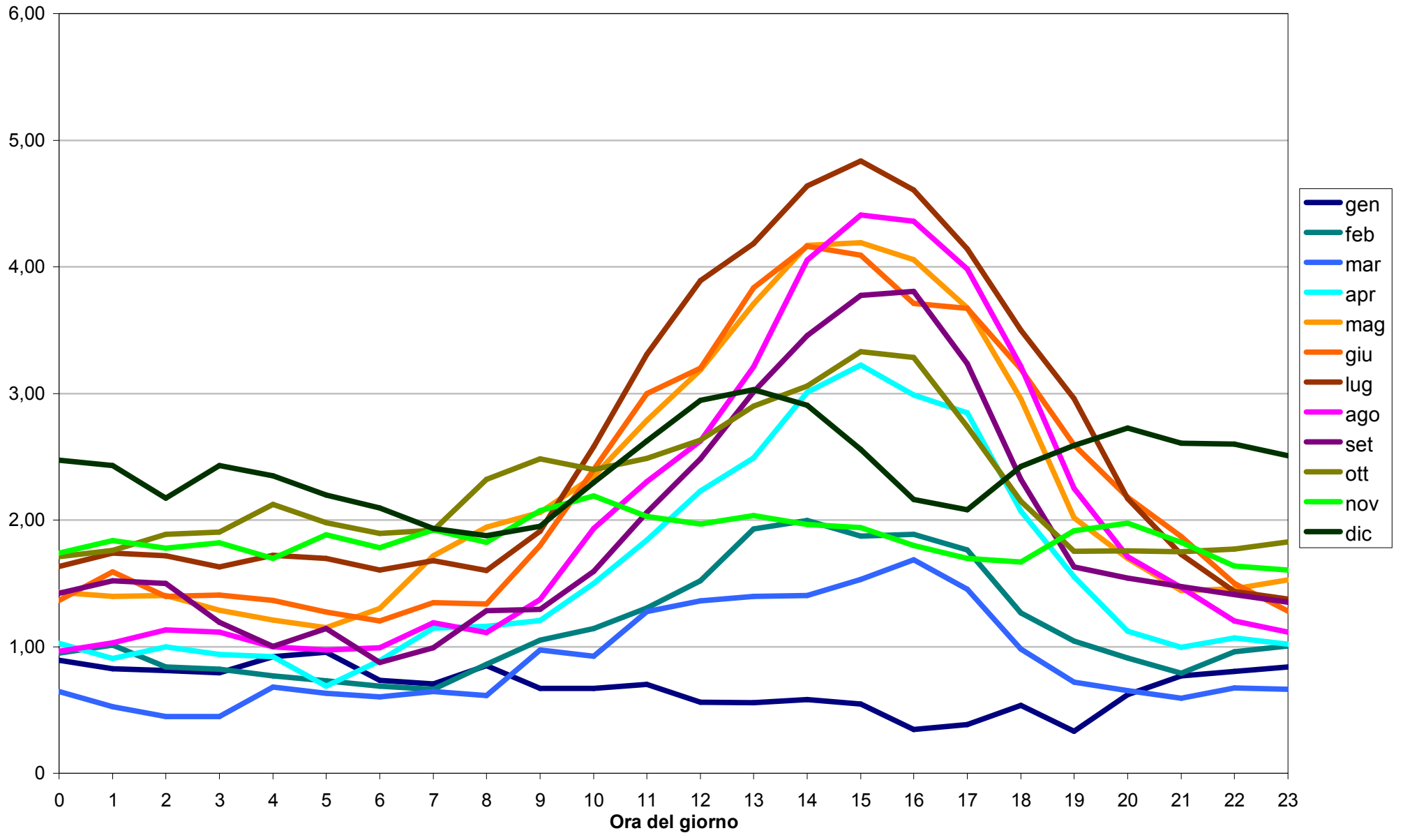
Allegato 3. Figura 3.02. Medie della velocità del vento media scalare oraria (in m/s), secondo il mese e l'ora.
