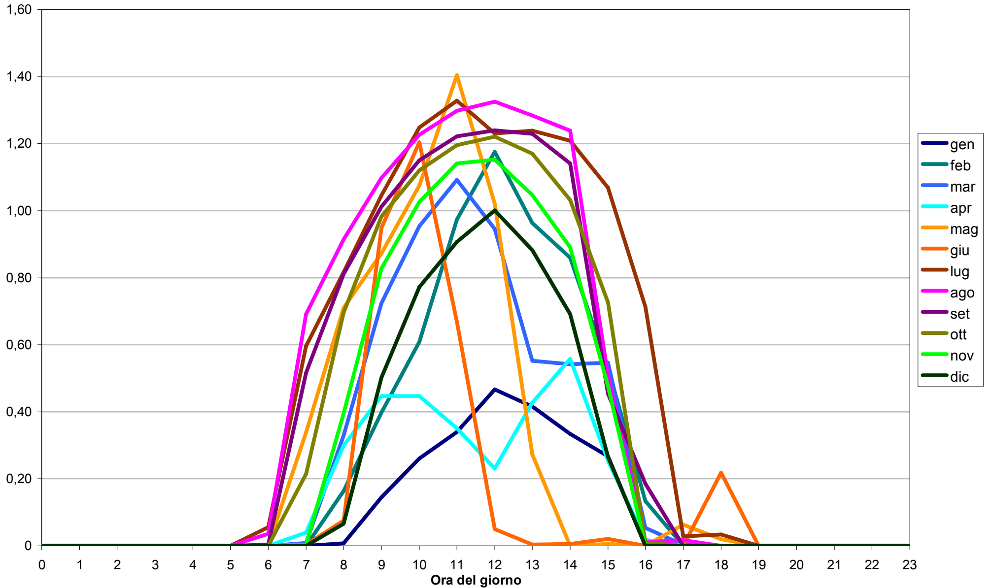
Allegato 3. Figura 3.10. Medie della velocità di scala convettiva oraria (in m/s), secondo il mese e l'ora.
