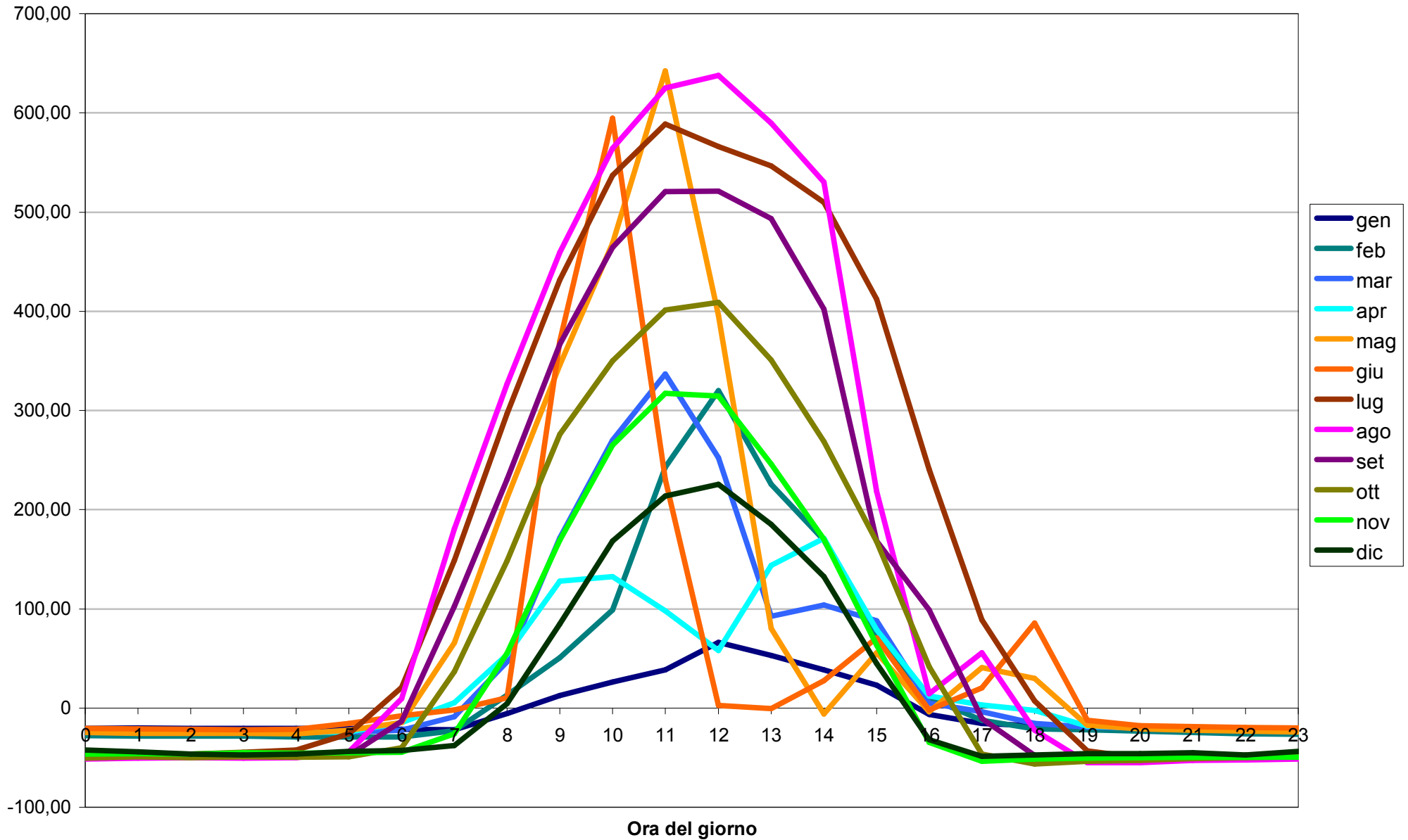
Allegato 3. Figura 3.05. Medie della radiazione solare netta oraria (in W/m 2 ), secondo il mese e l'ora.
