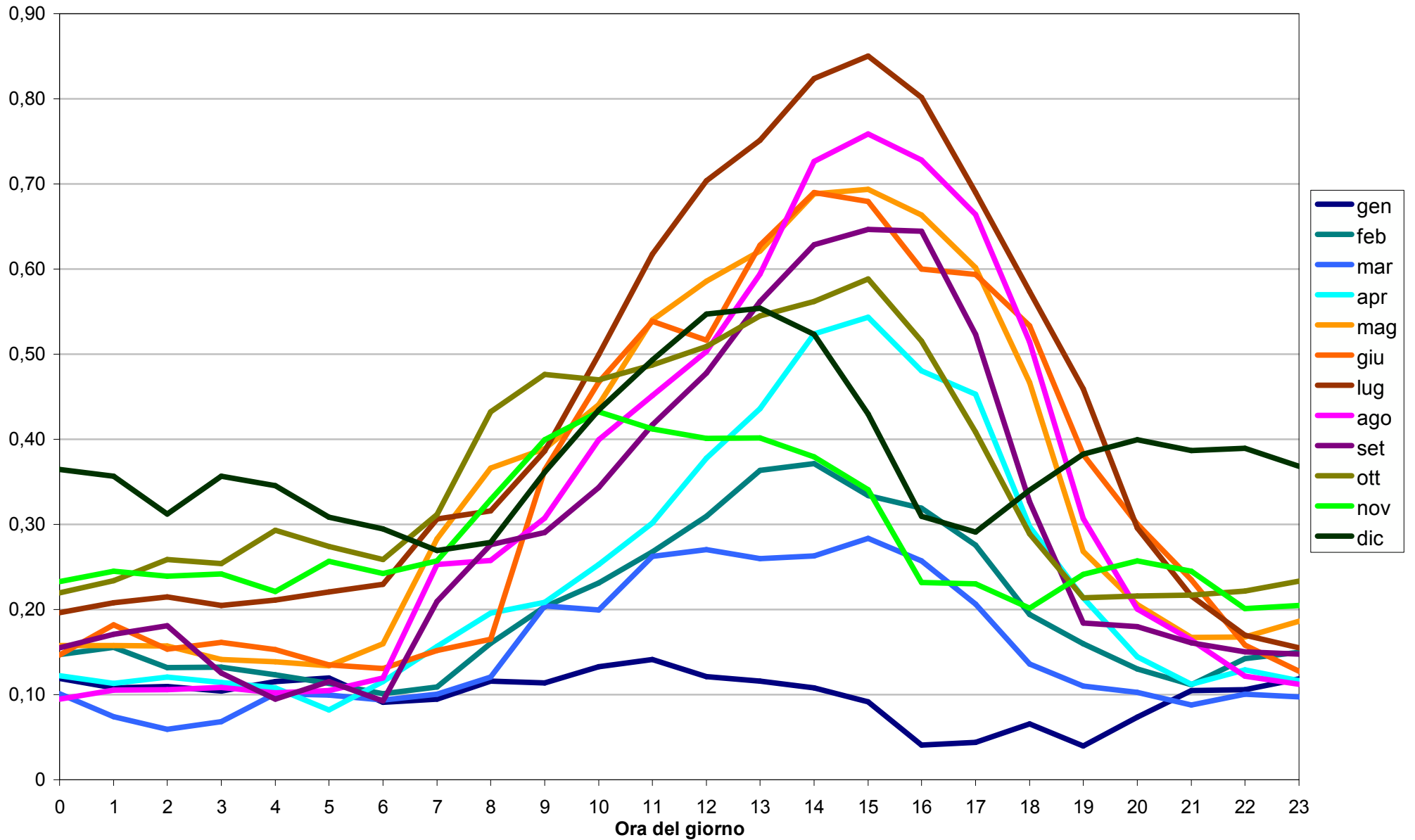
Allegato 3. Figura 3.07. Medie della velocità di attrito superficiale oraria (in m/s), secondo il mese e l'ora.
