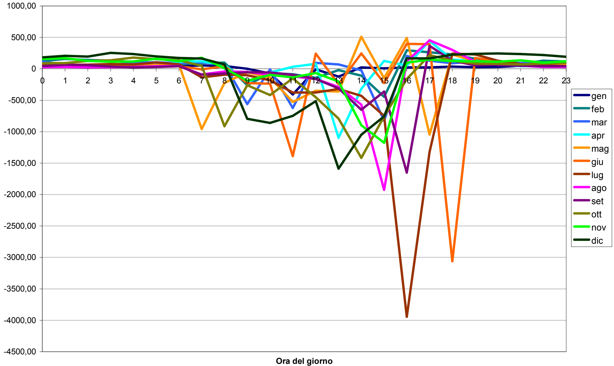
Allegato 3. Figura 3.06. Medie della Lunghezza di Monin-Obukhov oraria (in m), secondo il mese e l'ora.
