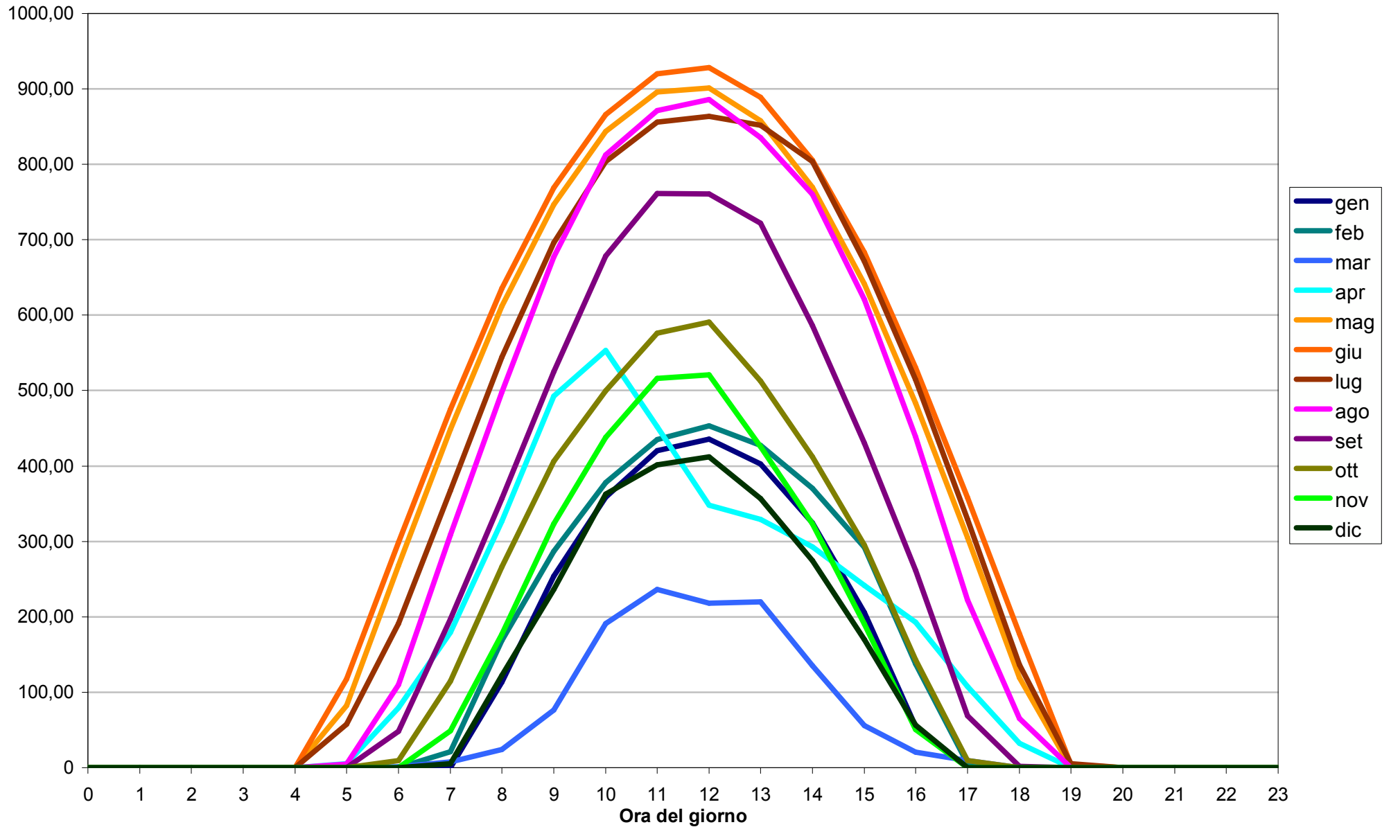
Allegato 3. Figura 3.03. Medie della radiazione solare globale oraria (in W/m 2 ), secondo il mese e l'ora.
