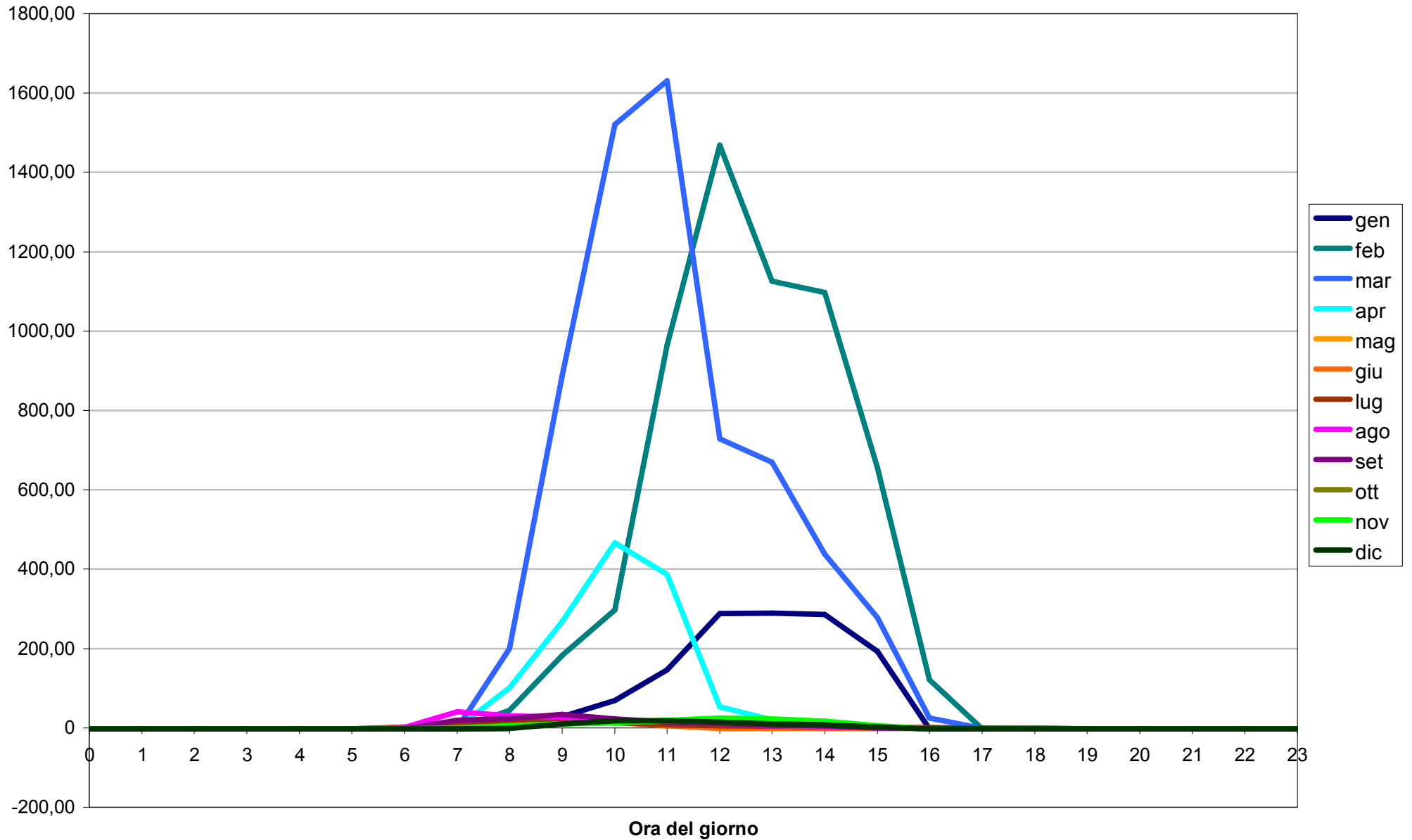
Allegato 3. Figura 3.11. Medie del rapporto -h/L orario (adimensionale), secondo il mese e l'ora.
