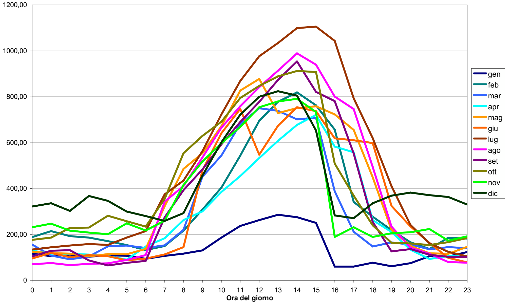
Allegato 3. Figura 3.09. Medie dell'altezza di mescolamento oraria (in m), secondo il mese e l'ora.
