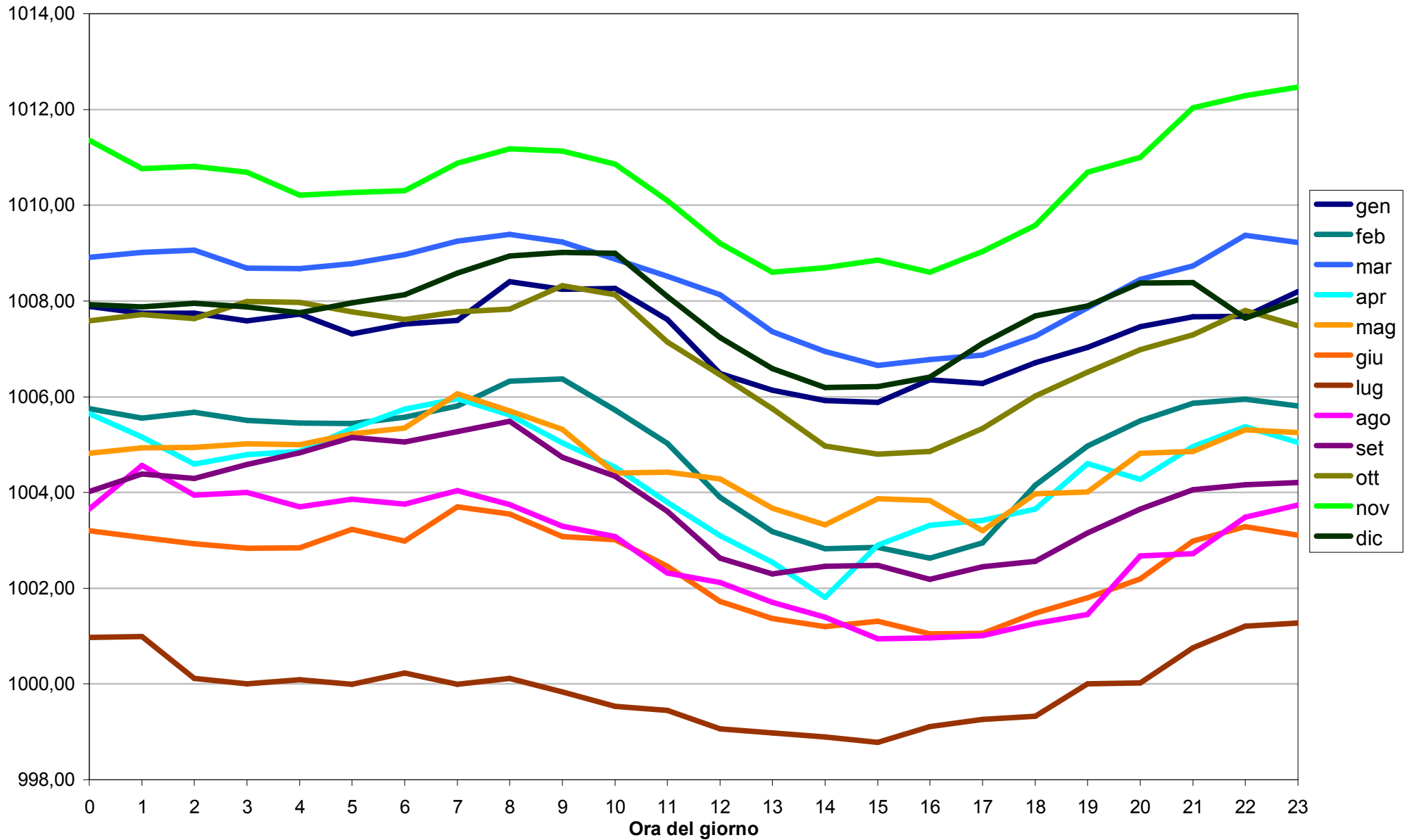
Allegato 3. Figura 3.04. Medie della pressione atmosferica oraria (in hPa), secondo il mese e l'ora.
