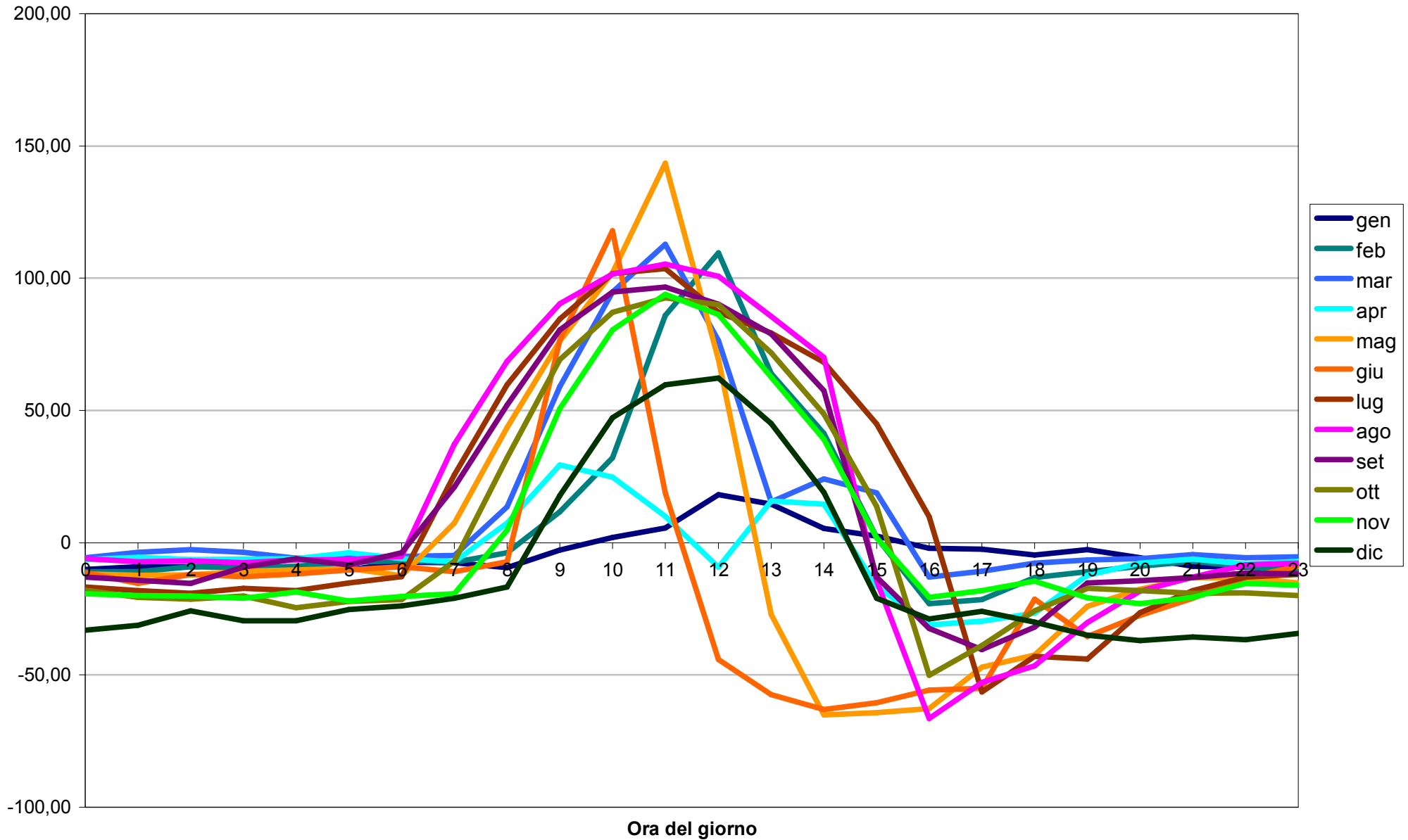
Allegato 3. Figura 3.08. Medie del flusso di calore sensibile superf. orario (in W/m 2 ), secondo il mese e l'ora.
