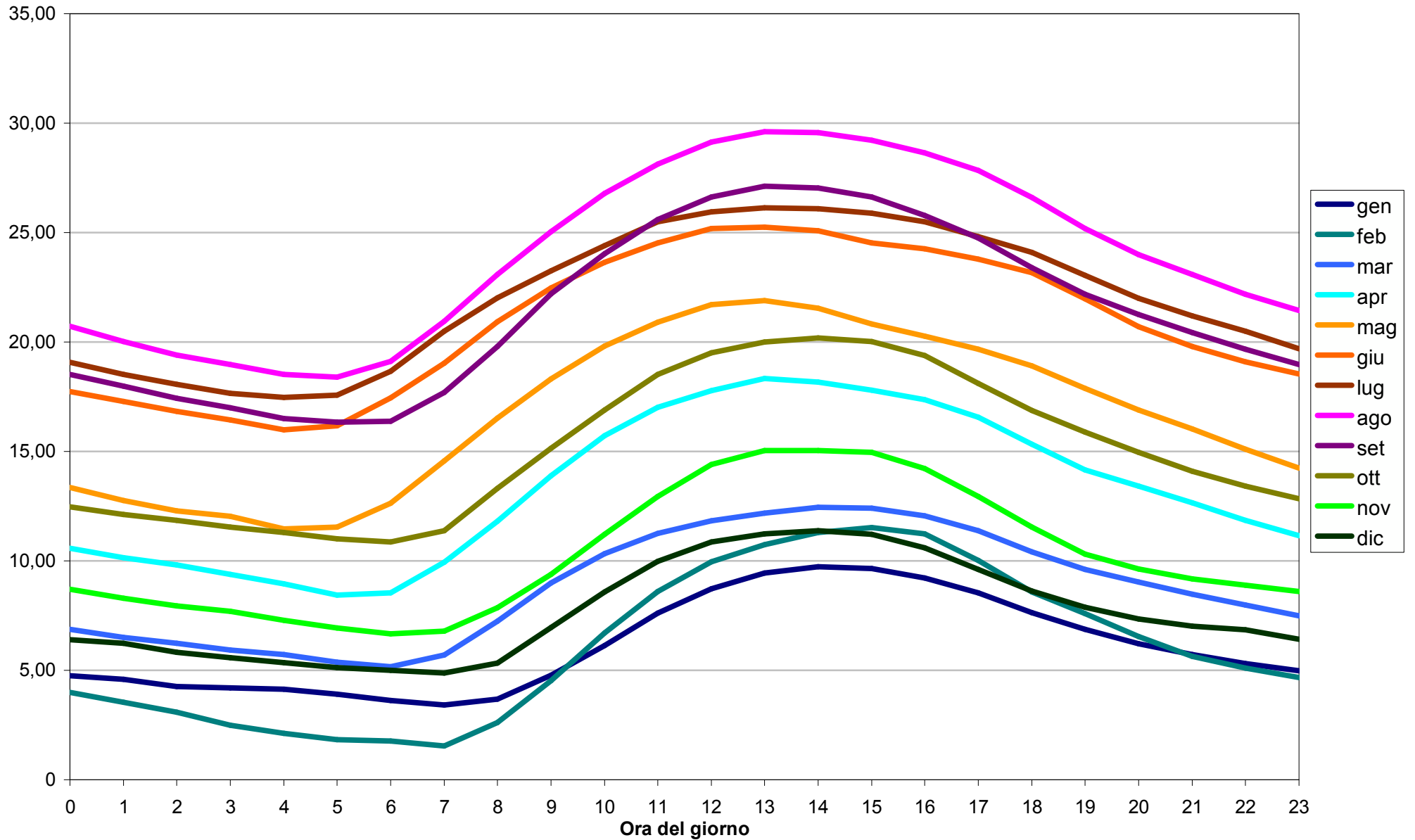
Allegato 3. Figura 3.01. Medie della temperatura dell'aria oraria (in °C), secondo il mese e l'ora.
