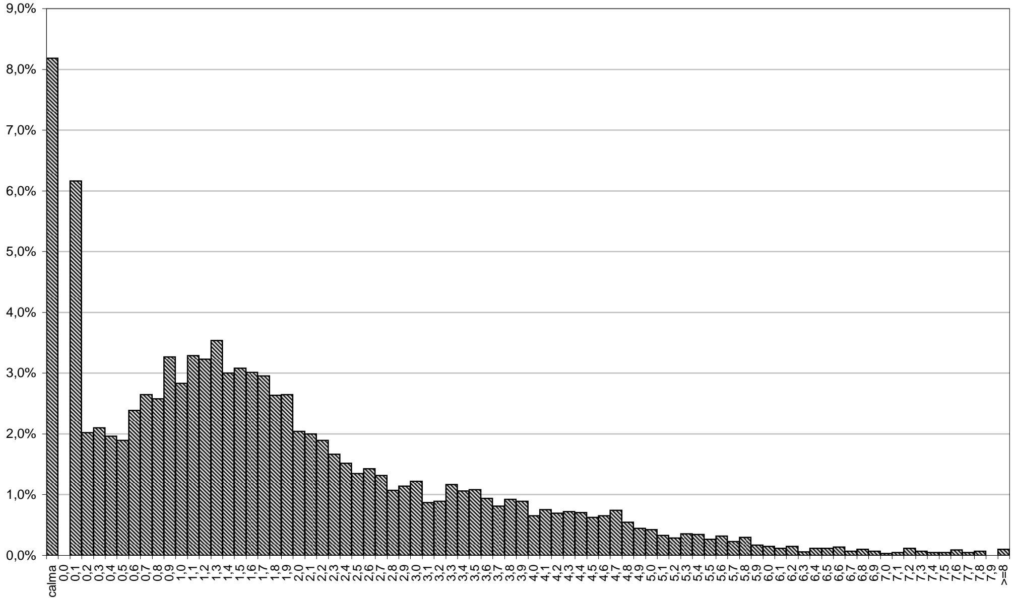
Allegato 5. Figura 5.01. Distribuzione della velocità del vento oraria (in m/s).
