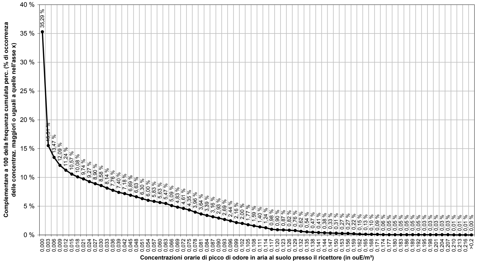
Allegato 7. Figura 7.02. Complementare a 100 della frequenza cumulata percentuale annua delle concentrazioni orarie di picco di odore presso il ricettore 2
