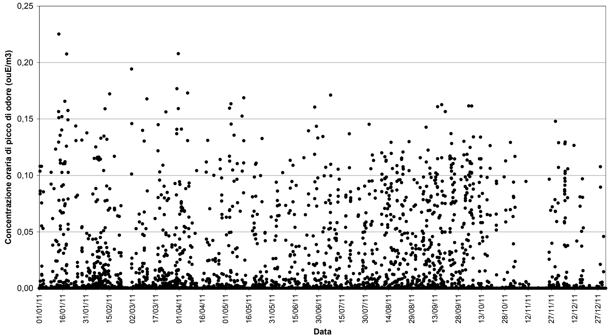
Allegato 7. Figura 7.03. Serie completa dei risultati delle simulazioni presso il ricettore 2
